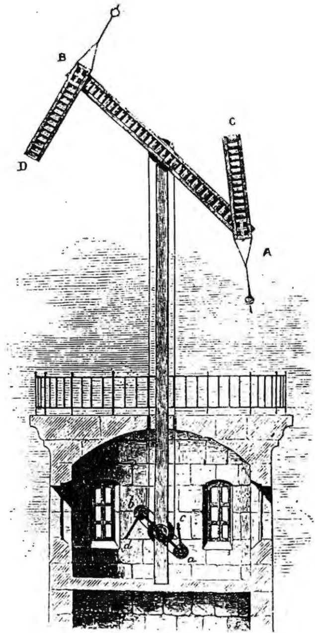
Principes du Semaphore Chappe.
